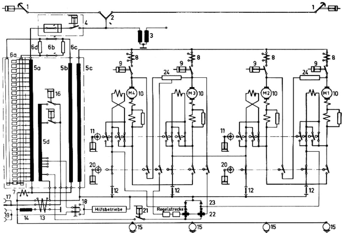
Prinzipialschaltplan Lok E 10
